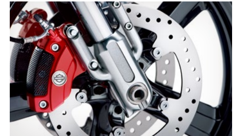
ブレーキキャリパーキット/レッド&ポリッシュブレーキローター
