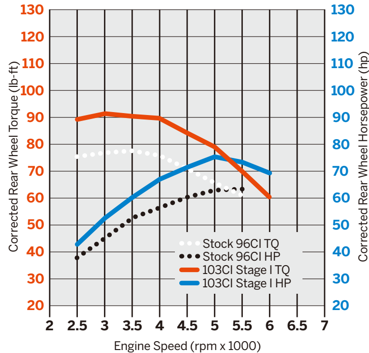
TWIN-CAM96(ノーマル) VS. 103ステージIキット
