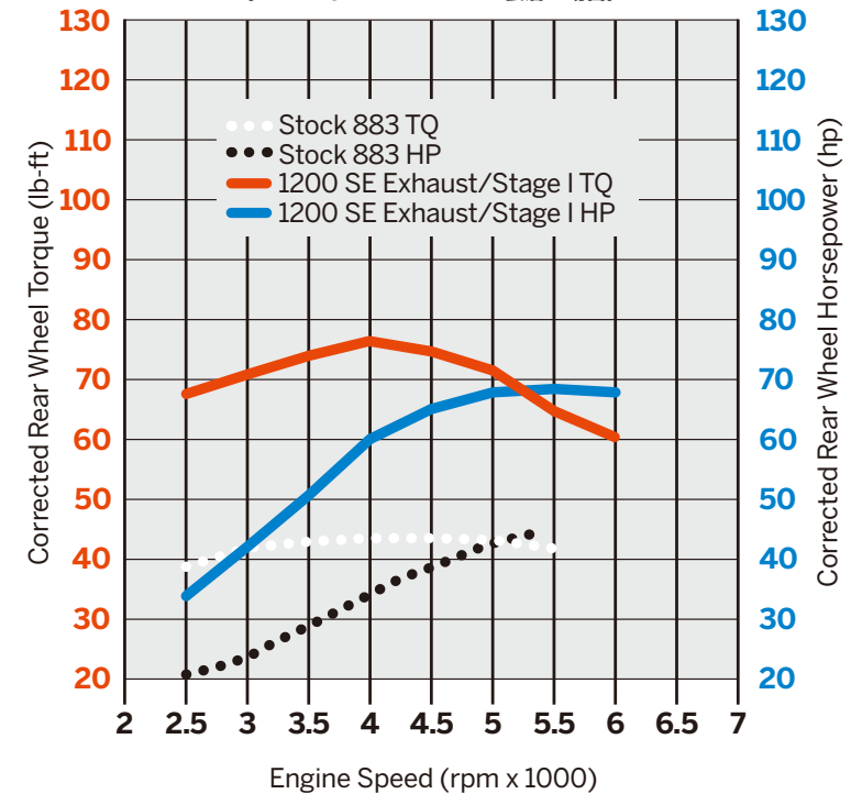
スポーツスター883(ノーマル) vs. 1200ステージIキット (SEパフォーマンスマフラー装着の場合)
