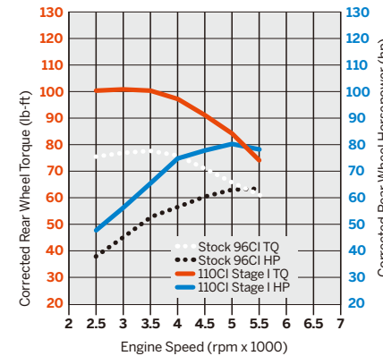
TWIN-CAM96(ノーマル) VS. 110ステージIキット
