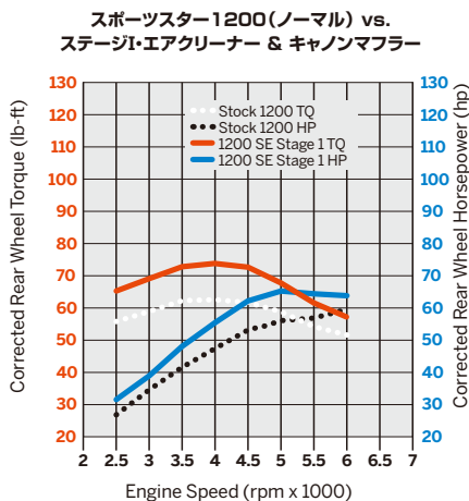
B スクリーミンイーグル・スポーツスター・ステージI・エアクリナーキット / オーバル
