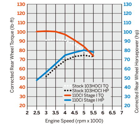
TWIN-CAM103(ノーマル) VS. 110ステージIキット
