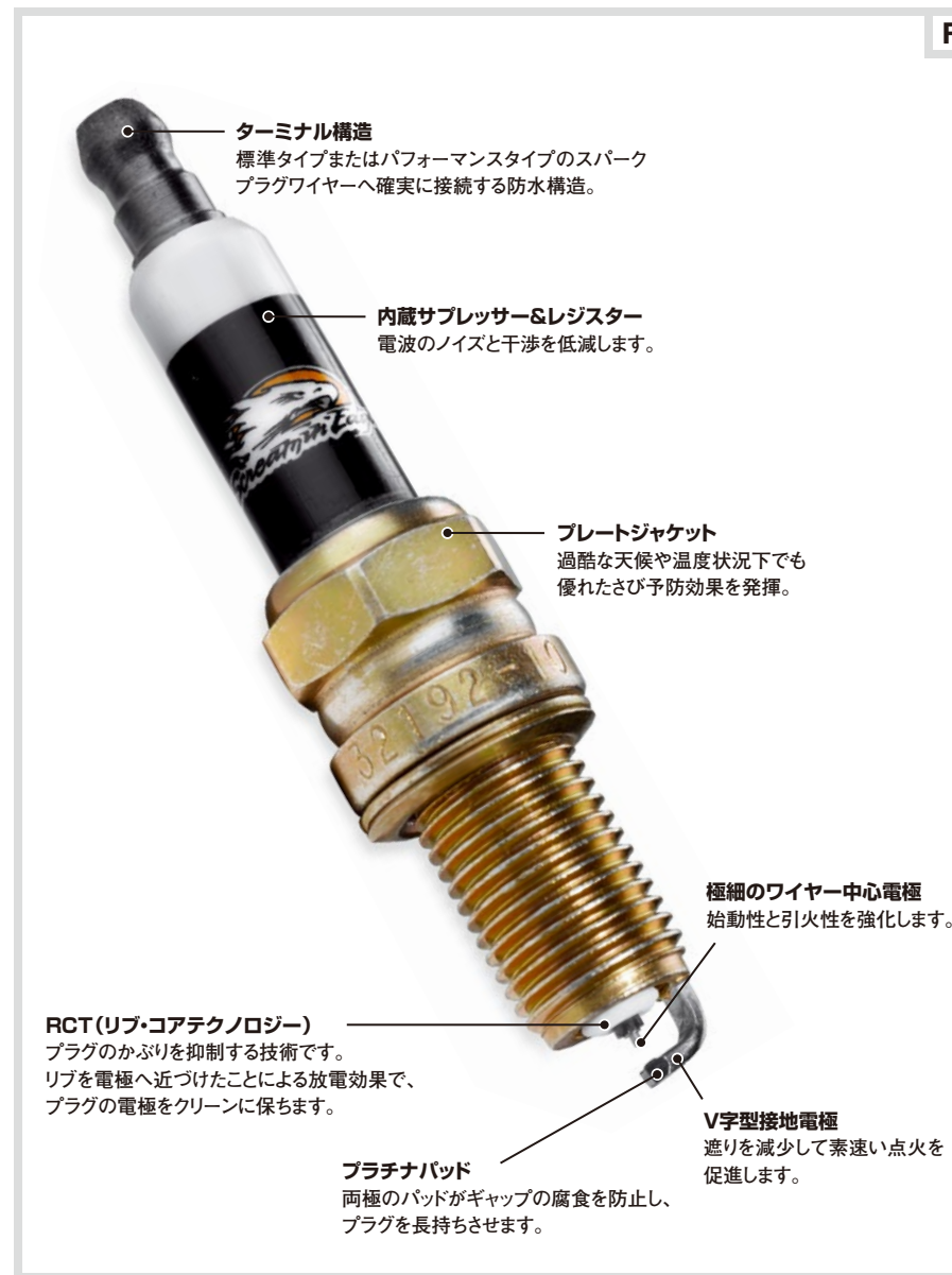
F スクリーミンイーグルST・パフォーマンス・スパークプラグ
